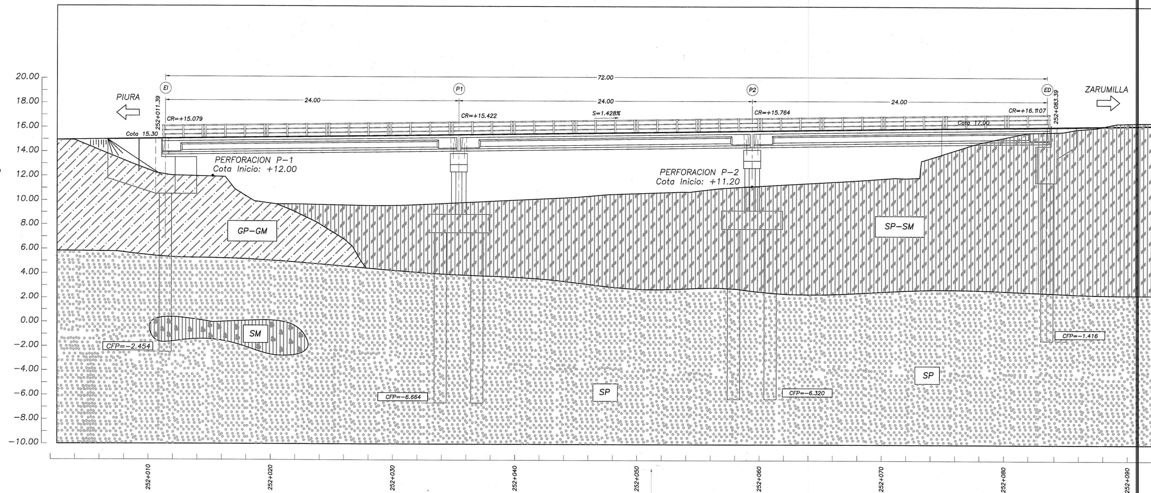
PERFIL ESTRATIGRAFICO Y REGISTRO DE PERFORACIONES P1 y P2 ESC:1/300
