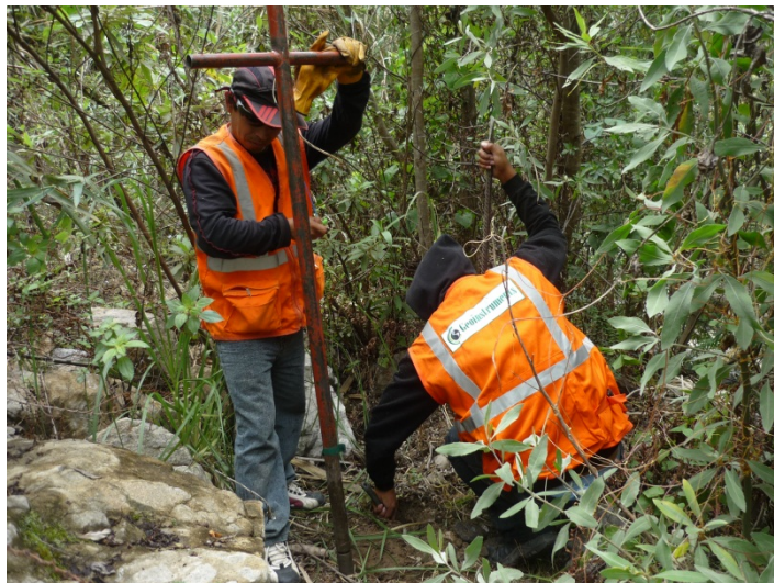
Foto 08.- Vista de la instalación de la Escopeta Sísmica para la Línea L-04.
